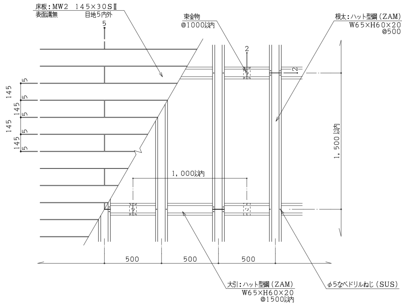
平面図 S=1:20
