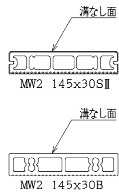
断面図 S=1:5
