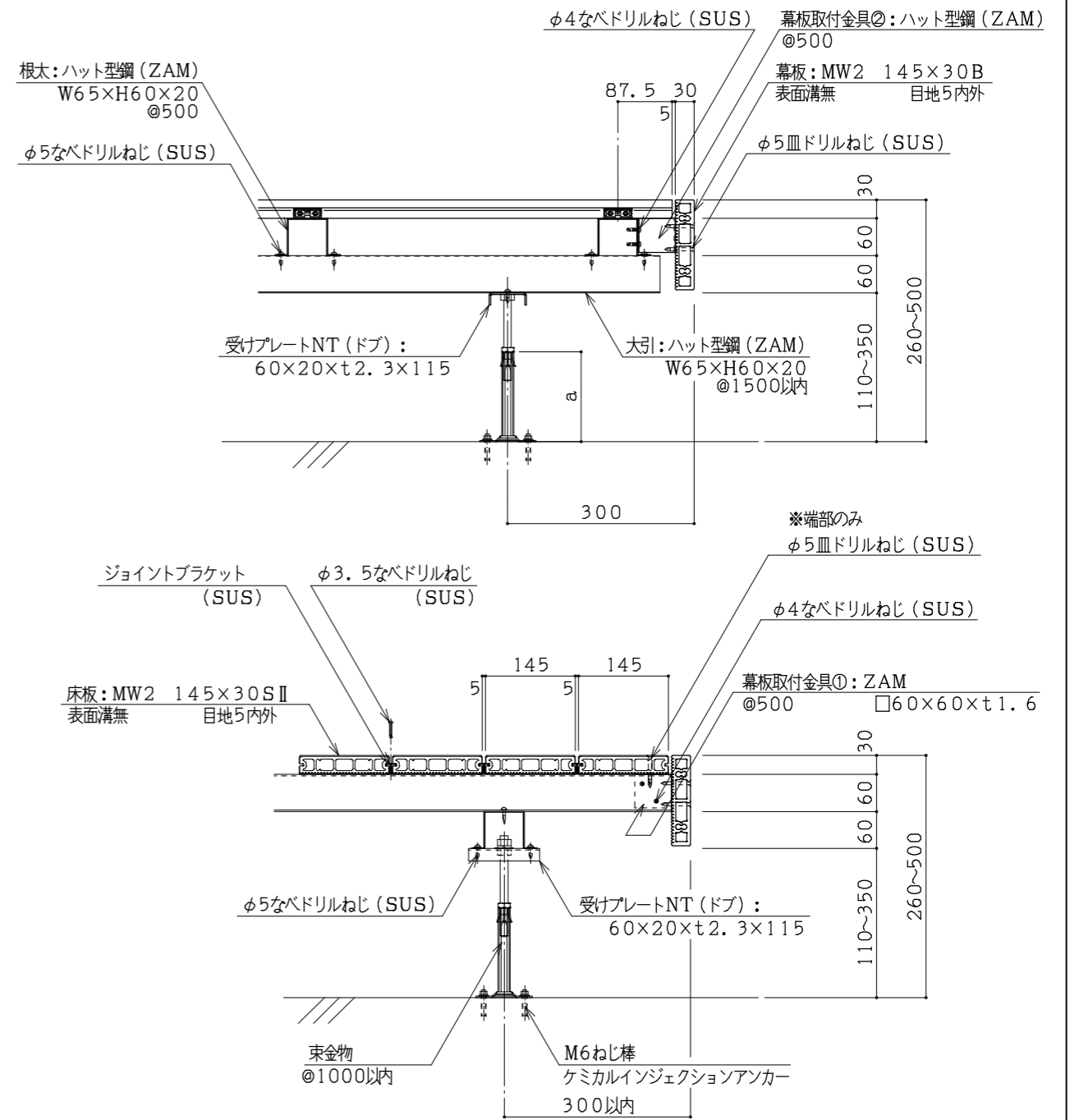
断面図 S=1:10
