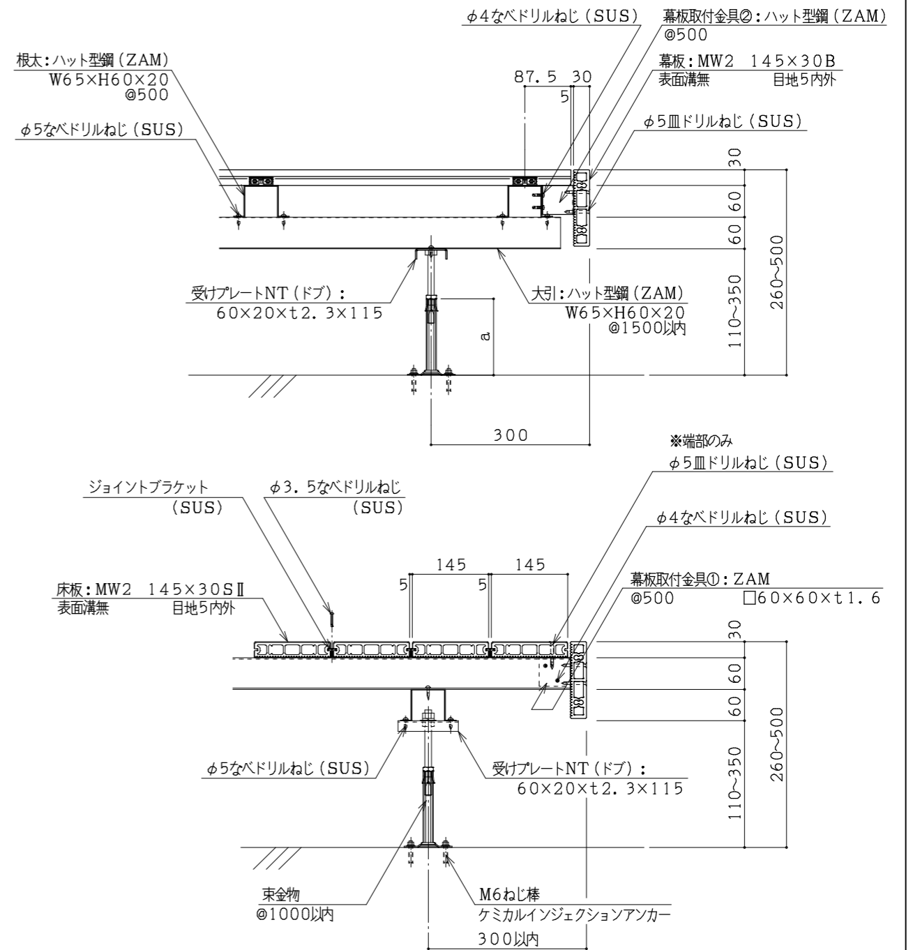
断面図 S=1:10
